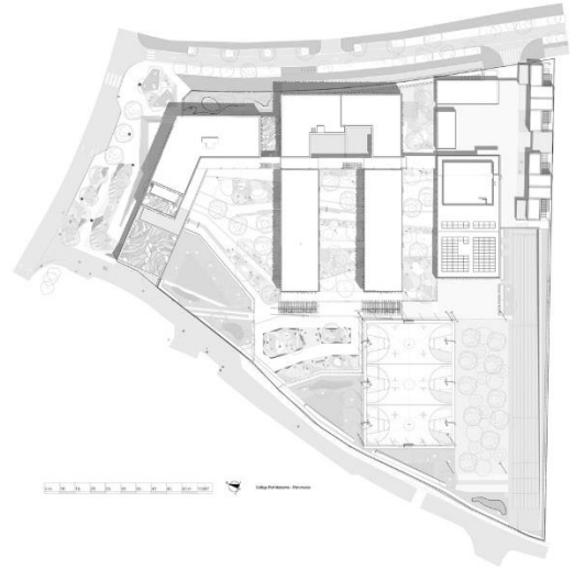
Helyszínrajz
