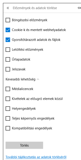
Edge
